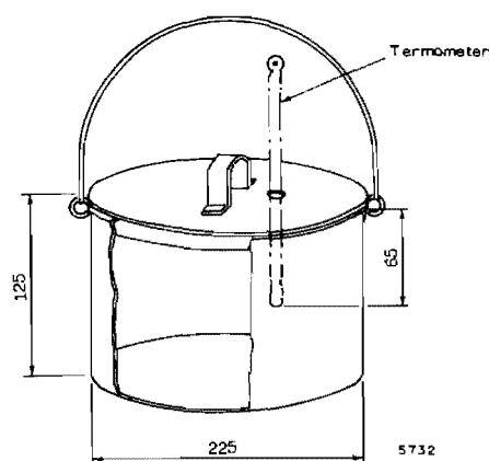
Fig. 1 - Kookapparaat
