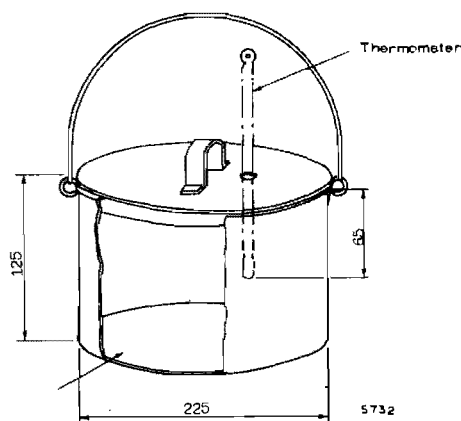
Fig. 1 - Cooking Utensil
