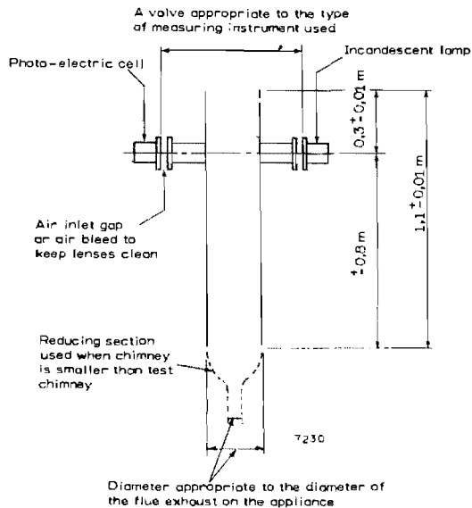
Fig. 3 - Test Chimney
