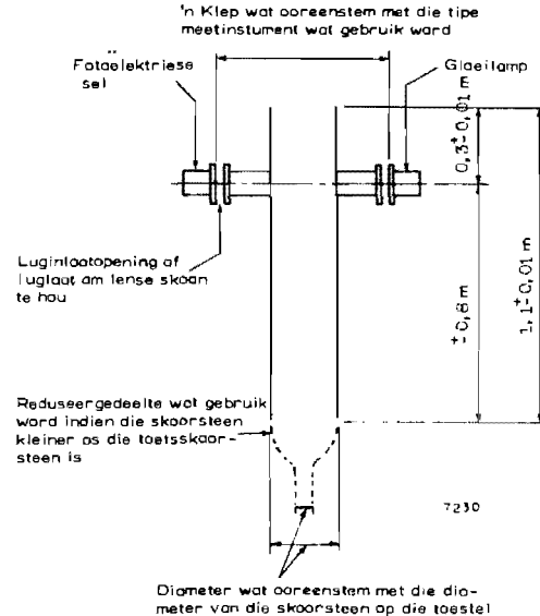
Fig. 3 - Toetskooorsteen
