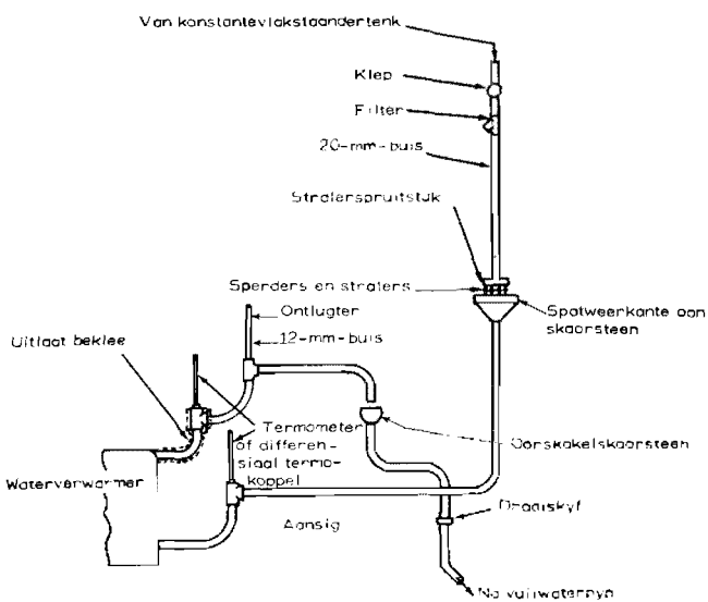
Fig. 2 - Tiese Watertoevoerverbindings vir Toets
